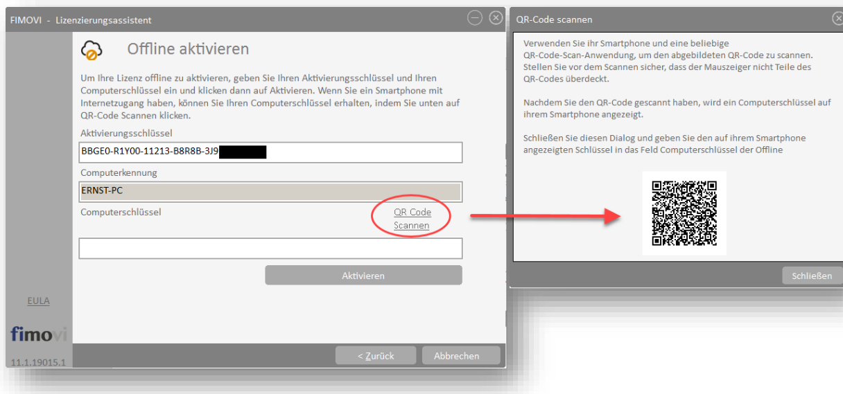
Abb. 1.8: Offline-Aktivierung - Eingabe Aktivierungsschlüssel und Computerschlüssel
